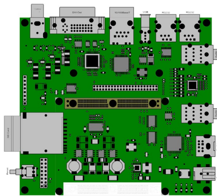
CRX03 - Oberseite
